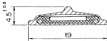
A-A断面拡大図(S=3/1)
