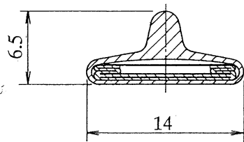
A-A断面拡大図 (S = 3/1)
